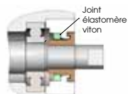
Rouleau haute température 150°C Ambiance sidérurgie
