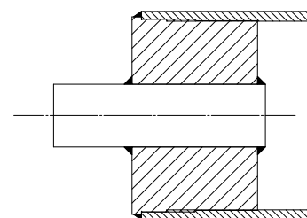
Tambour à tourillons
